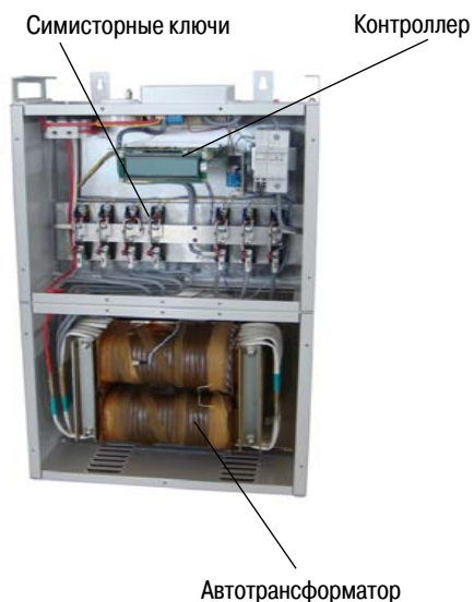
Рис. 8. Устройство стабилизатора
